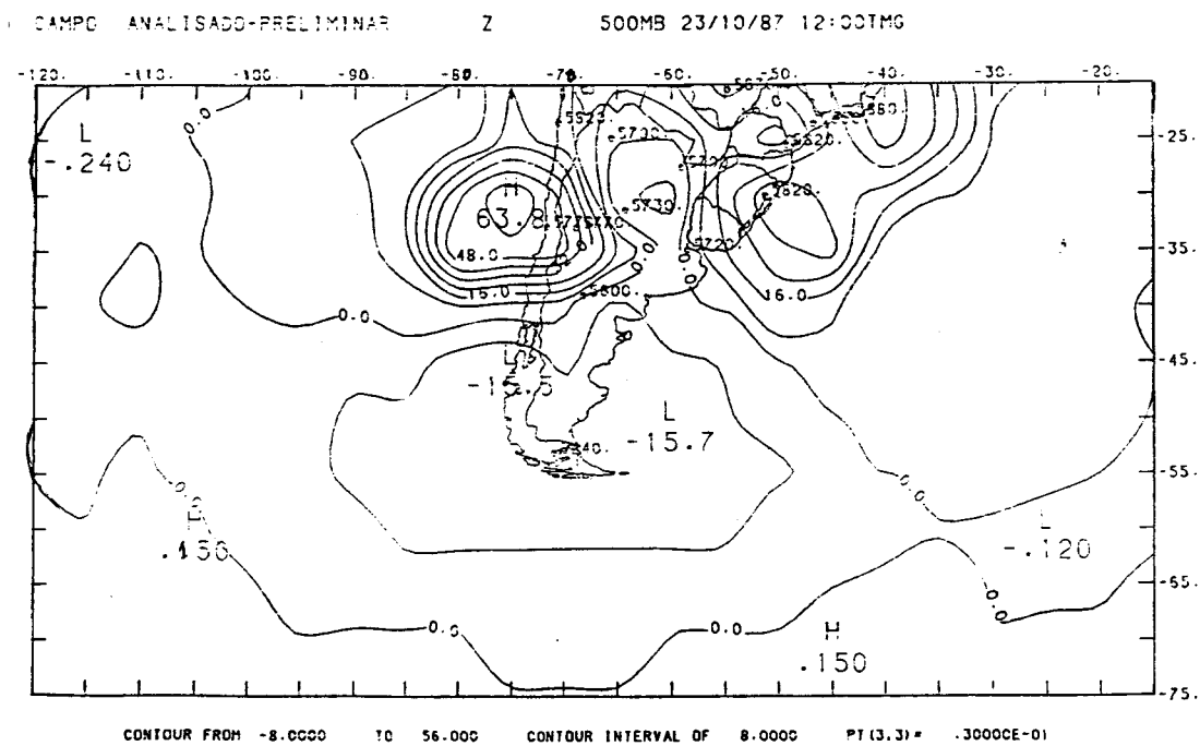
Fig. 5 - Campo de diferenças entre o campo analisado e o preliminar, para 500 mb, 23.10.87, 12:00 TMG.
